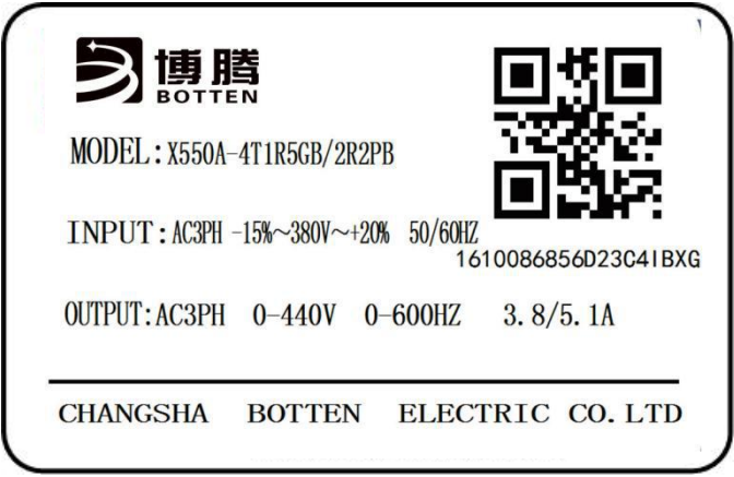
图2-2. 铭牌
