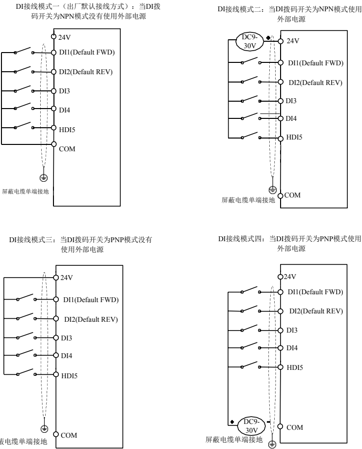
图3-6. 四种不同模式下数字输入端子接线图一
