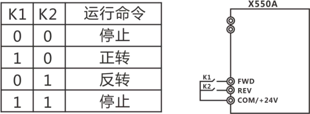
图5-1两线式运转模式1
