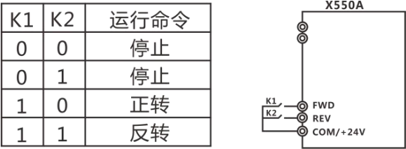
图5-2 两线式运转模式2
