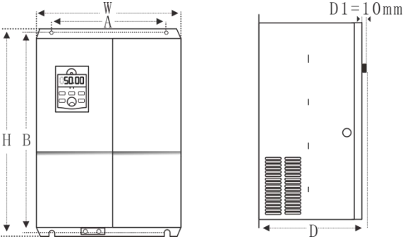
11-355kw外形尺寸
