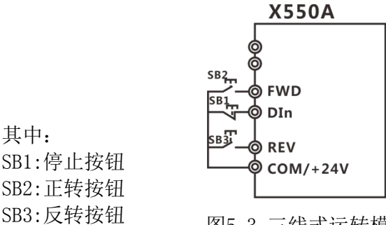
图5-3 三线式运转模式1
